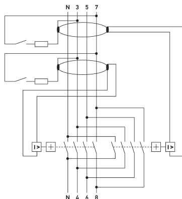
Anschlussschema
