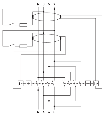
Anschlussschema
