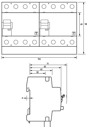
Maßzeichnung Gruppenansicht
