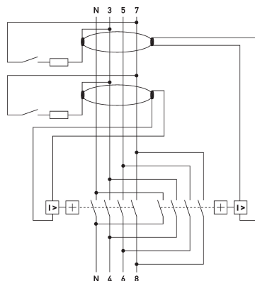
Anschlusschema
