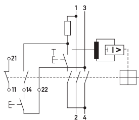
Anschlusschema
