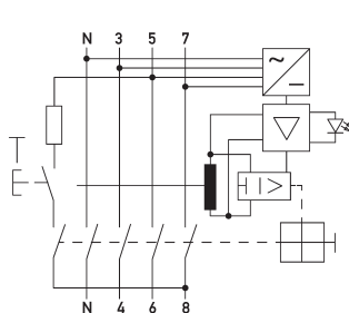
Anschlusschema
