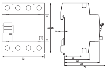
Maßzeichnung Gruppenansicht
