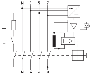
Anschlussschema
