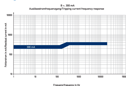
Kennlinie B+ 300 mA
