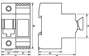
Maßzeichnung Gruppenansicht
