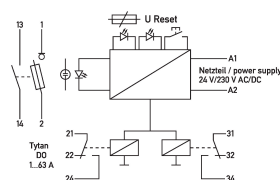
Anschlusschema
