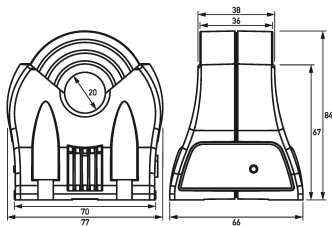
Maßzeichnung Gruppenansicht
