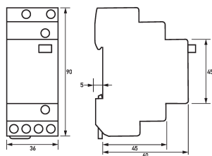
Maßzeichnung Gruppenansicht
