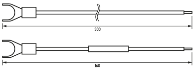
Maßzeichnung Gruppenansicht
