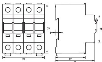
Maßzeichnung Gruppenansicht
