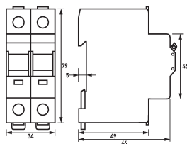
Maßzeichnung Gruppenansicht
