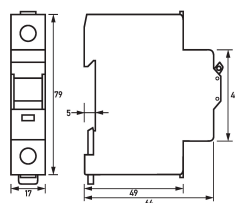
Maßzeichnung Gruppenansicht
