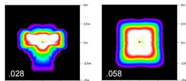
asymmetrisch breitstrahlend Höhe: 800mm; Fläche: 10m x 10m
