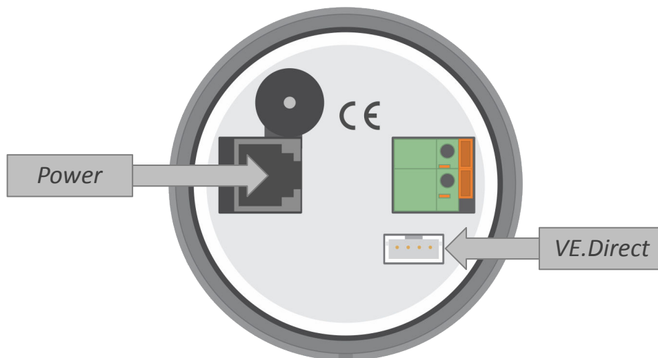
Auf der Rückseite des MPPT Control befinden sich der Stromanschluss und der VE.Direct-Anschluss
