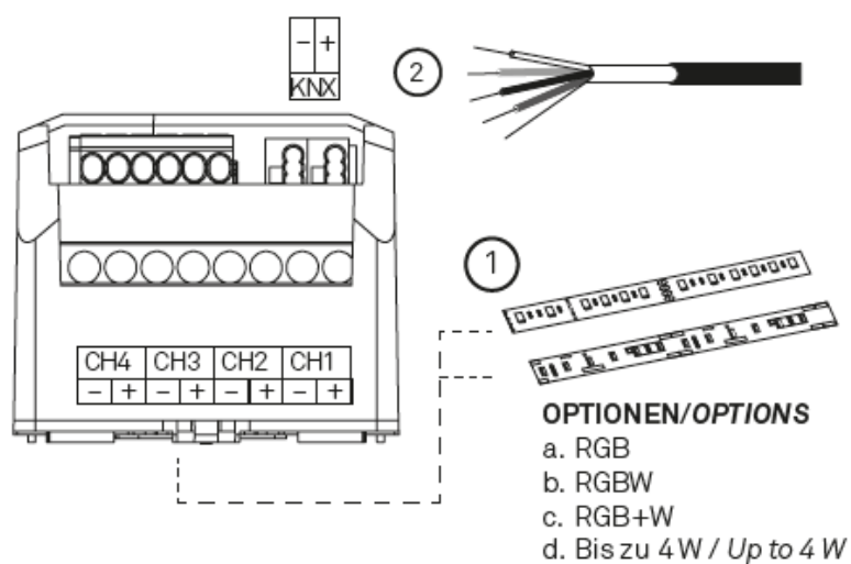
Abbildung 9: Anschluss Ausgänge
