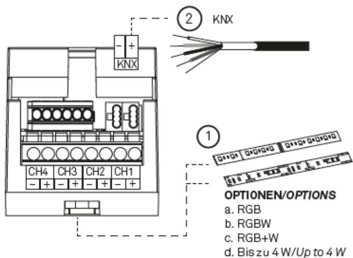
Abbildung 6: Anschluss Ausgänge
