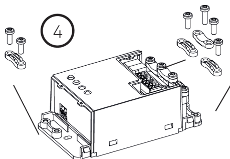
Abbildung 4: Kabel-Zugentlastungen
