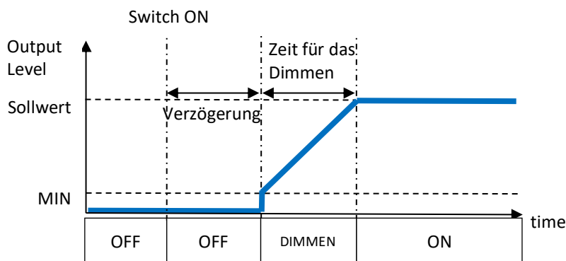
Abbildung 35: Verzögerung beim Einschalten und Dimmen zum Sollwert
