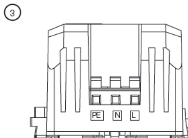
Abbildung 10: Anschluss Versorgungsspannung
