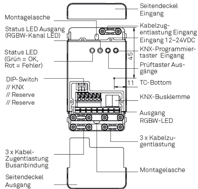
Abbildung 1: Gerätebeschreibung KNX LED-Dimmer BASIC
