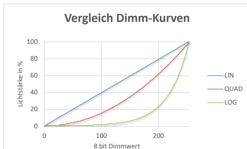
Abbildung 16: Vergleich Dimm-Kurven
