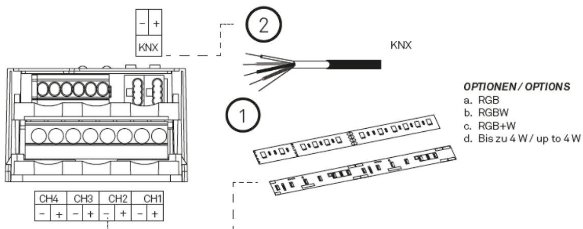
Abbildung 2: Anschluss Ausgänge
