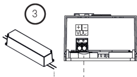
Abbildung 3: Anschluss Versorgungsspannung
