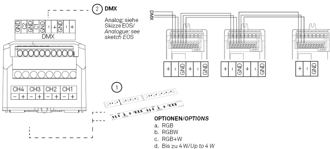
Abbildung 9: Anschluss Ausgänge
