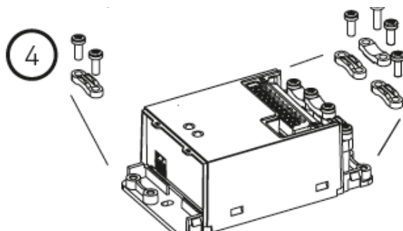
Abbildung 4: Kabel-Zugentlastungen
