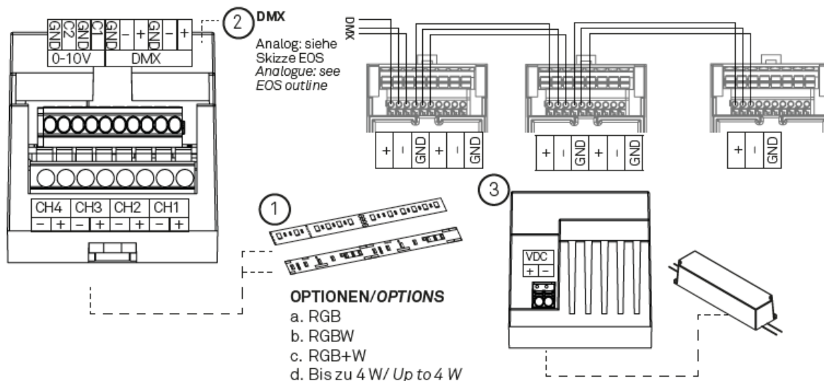
Abbildung 6: Anschluss Ausgänge
