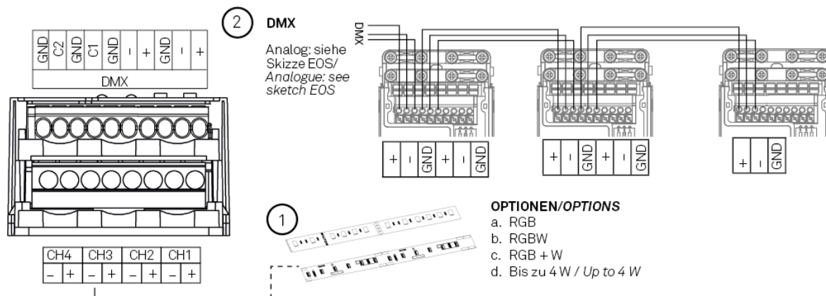
Abbildung 2: Anschluss Ausgänge
