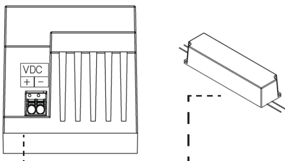
Abbildung 7: Anschluss Versorgungsspannung
