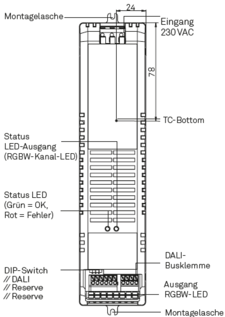
Abbildung 8: Gerätebeschreibung DALI LED-Dimmer SXT
