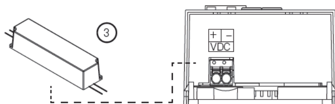
Abbildung 3: Anschluss Versorgungsspannung
