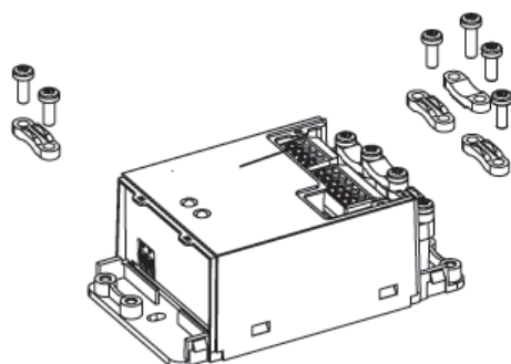
Abbildung 4: Kabel-Zugentlastungen
