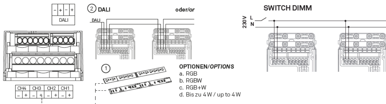
Abbildung 2: Anschluss Ausgänge
