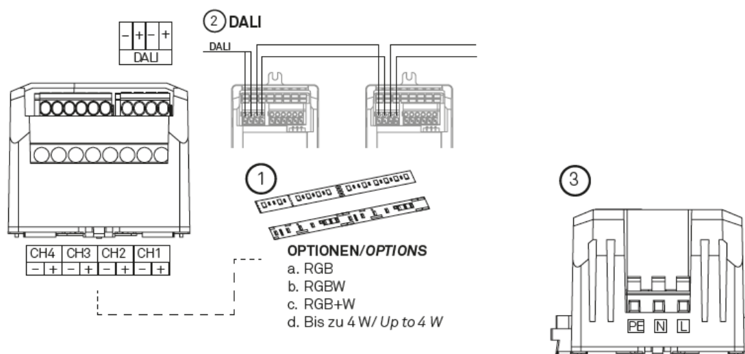
Abbildung 9: Anschluss Ausgänge/ Versorgungsspannung
