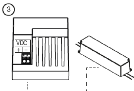
Abbildung 7: Anschluss Versorgungsspannung
