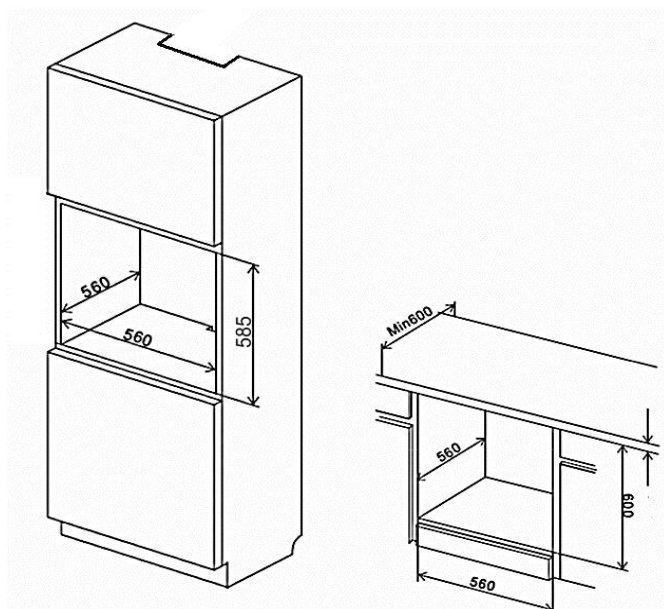
Einbauskizze
