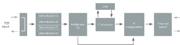
Blockdiagramm
