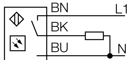
Anschlussbild
