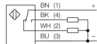
Anschlussbild
