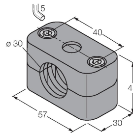
BSS-30
