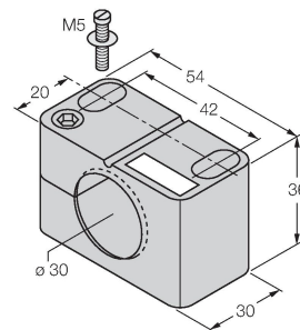
BSS-30
