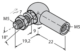
Winkelgelenk für geführte Positionsgeber; Material: Edelstahl
