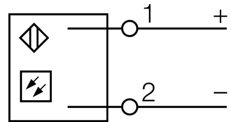
Anschlussbild
