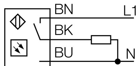
Anschlussbild
