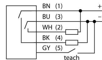
Anschlussbild
