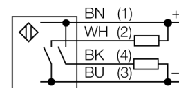
Anschlussbild
