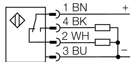
Anschlussbild
