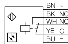
Anschlussbild
