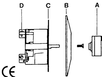
Seitenansicht
