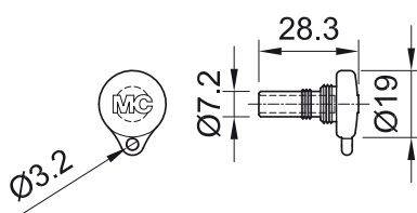
Stecker-Verschlusskappe (PV-SVK4)
