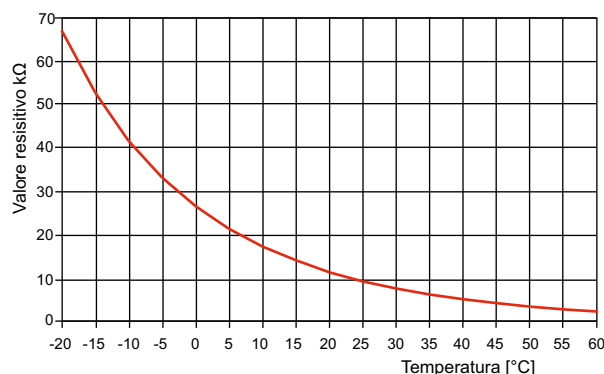
Fig. 7.3: Curva caratteristica della sonda NTC-10
