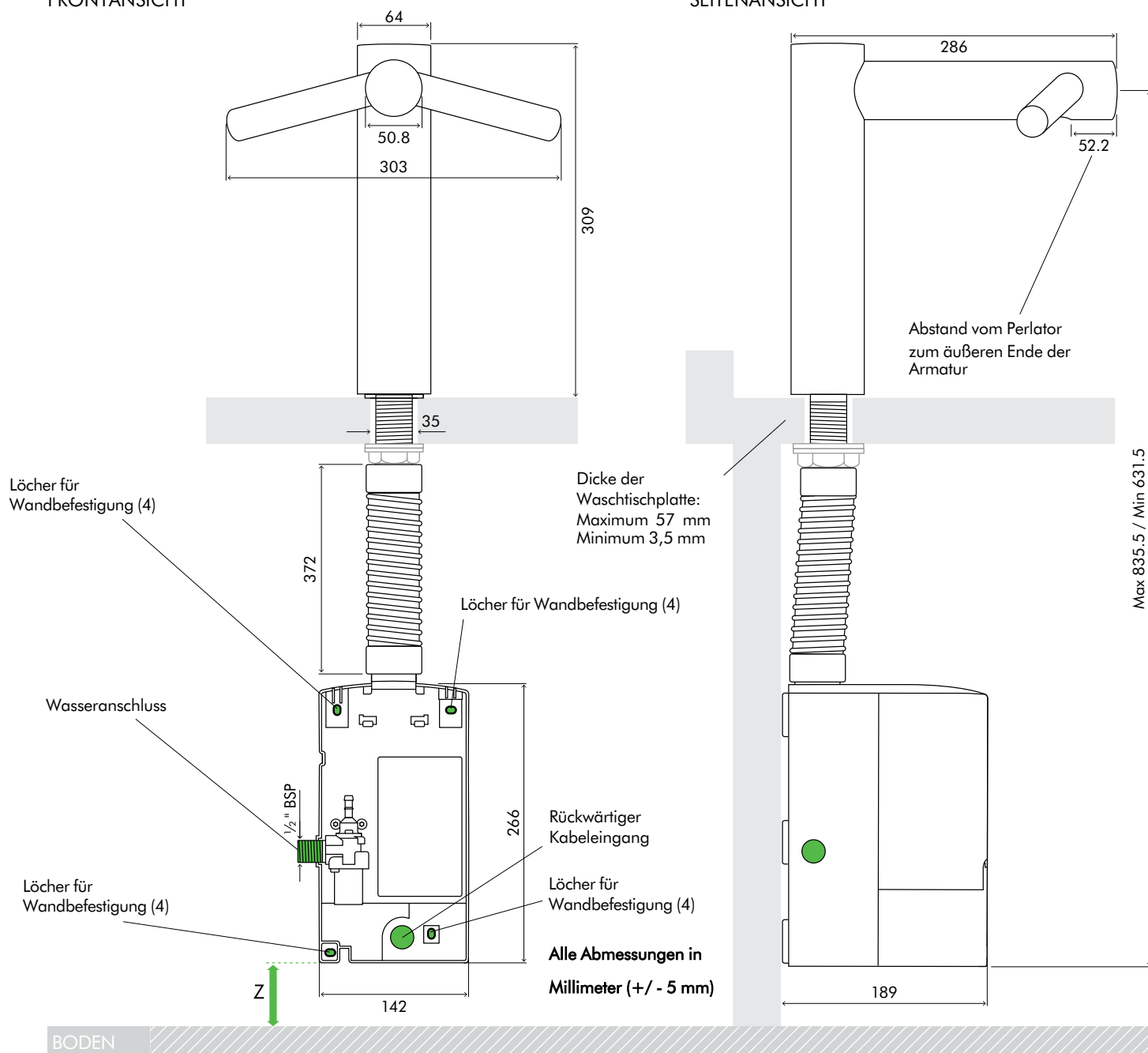
FRONTANSICHT
