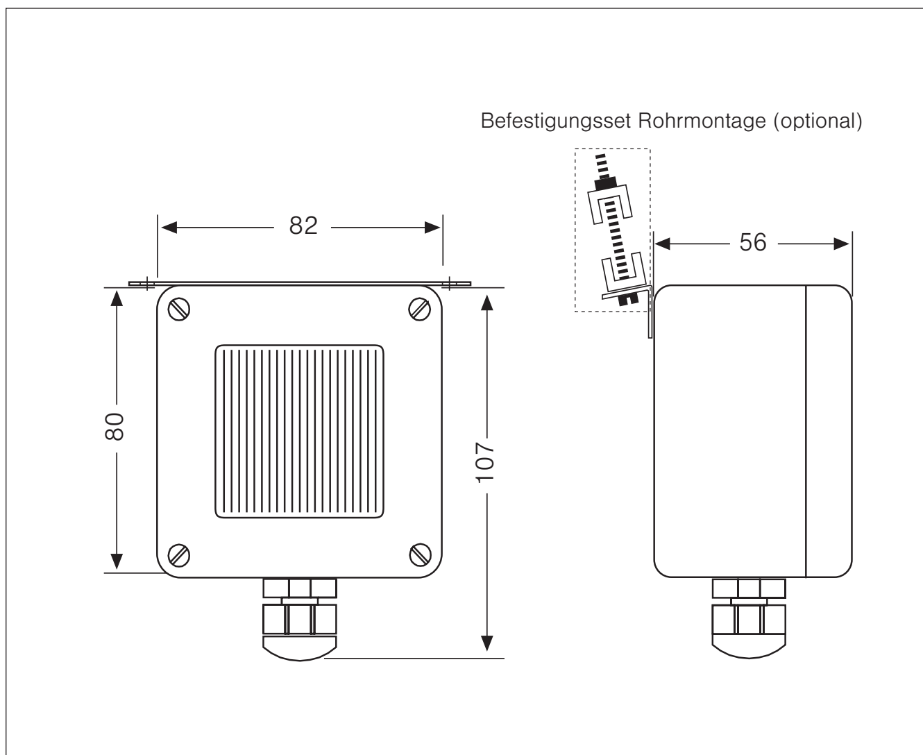
Abb. 2 Abmessungen
