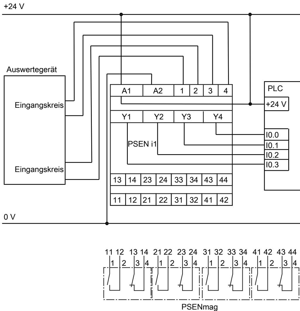
Abb.: Zweikanaliger Anschluss von vier PSENmag an den Eingangskreisen eines Auswertegeräts
