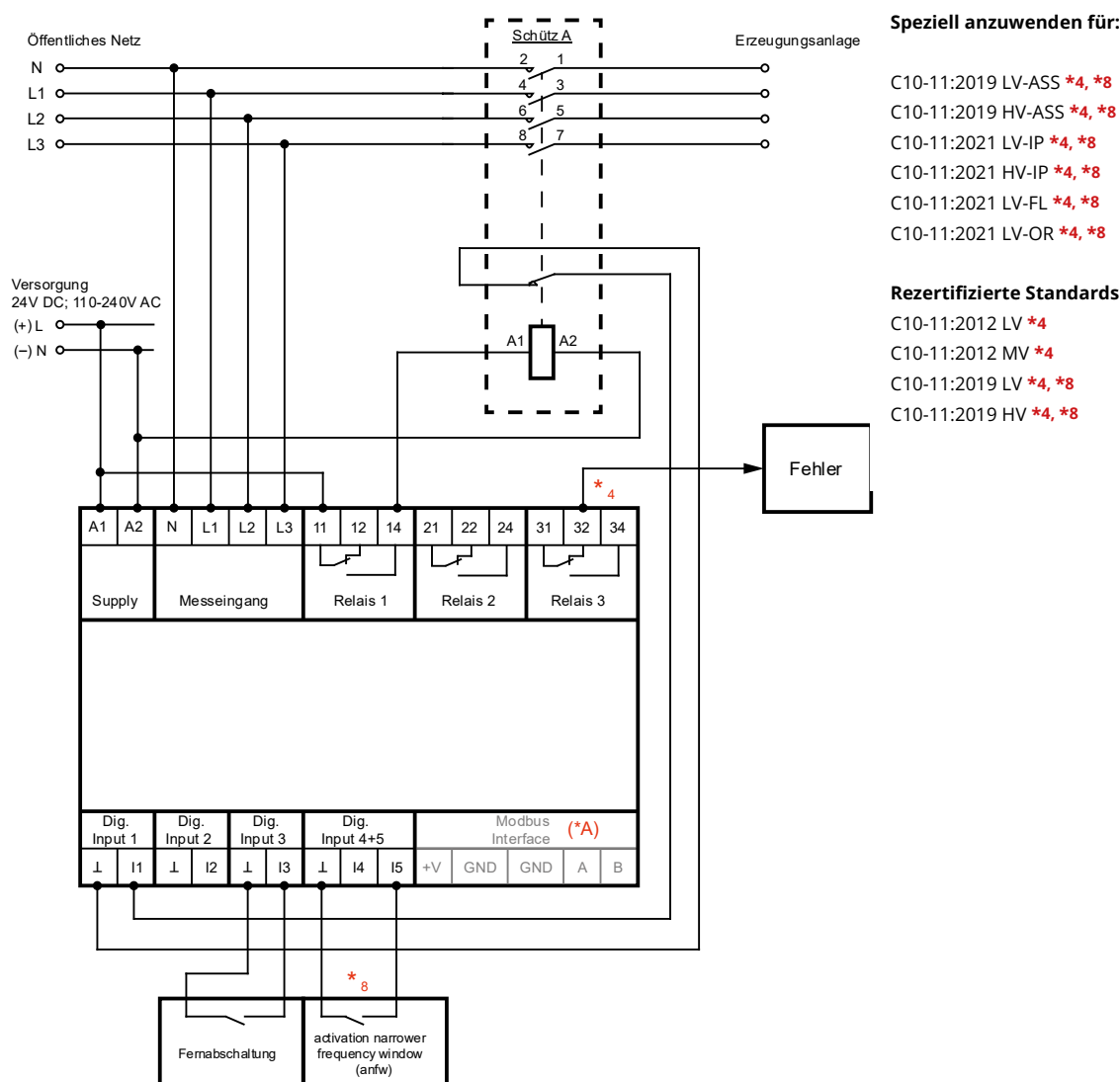
Abbildung 5: Anschlussbild 4 (C10/C11)
