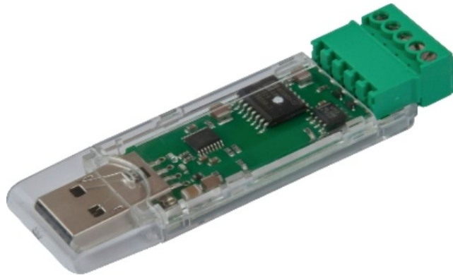
Abbildung 7: USB-to-RS485 Adapter, bestellbar auf www.tele-online.com mit der Bezeichnung S-USB485
