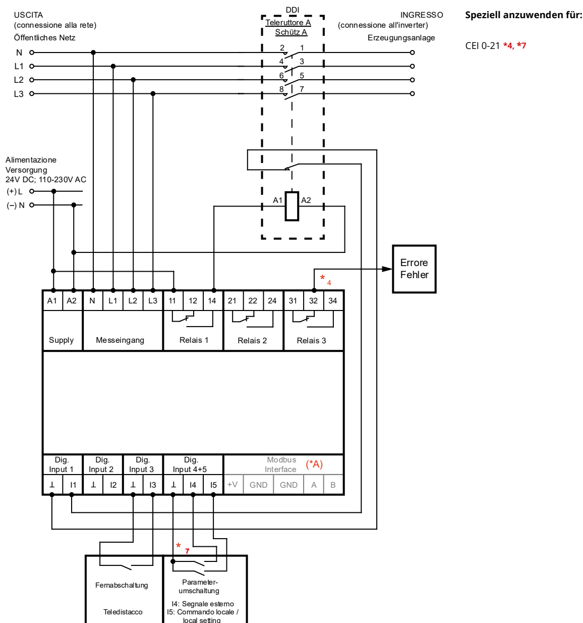
Abbildung 4: Anschlussbild 3 (CEI 0-21)
