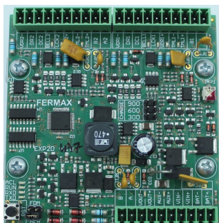
FERMAX AC-MAX KIT-Steuerplatine Erweiterung für 2 Türen
