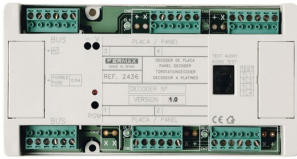
FERMAX MDS-Paneldecoder, 4 Ausgänge
