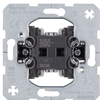
BERKER Wechselschalter Einsatz 10 A Up
