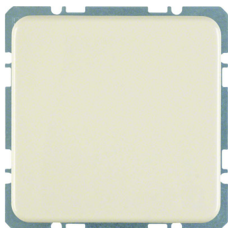
BERKER WG-UP SD NEMA5-20 R USA/CANADA Schutzkontakt, IP44, weiß glänzend
