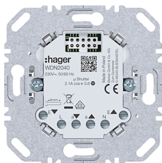
BERKER A.x/C.x Jalousie-Einsatz, 1fach UP
