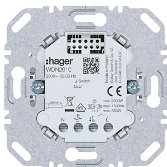
BERKER A.x/C.x Schalt-Einsatz, 1fach 10 A, Up
