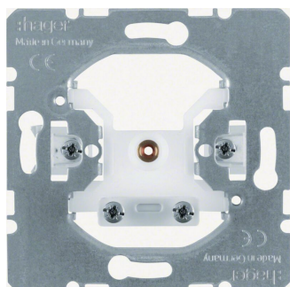
BERKER Kabelauslass, Zugentlastung ohne Klemmblock, UP
