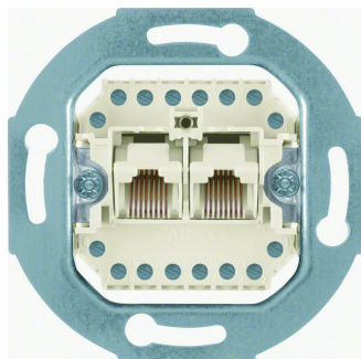
BERKER UAE-Steckdose 8/8-polig weiß
