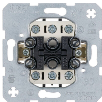
BERKER Wippenschalter 3 x 1-polig Aus mit Schraubklemmen
