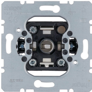
BERKER Drucktaster und Lichtsignal E10 Schließer, 2 A, UP
