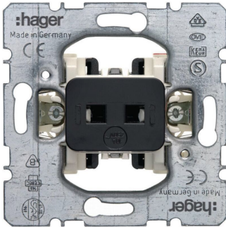
BERKER Wipptaster Hotelcard-Schließer Schalteraufsatz, 2 getr. Eingangskl., 10A
